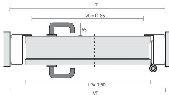
Corte Horizontal Horizontal cut Coupe horizontal
